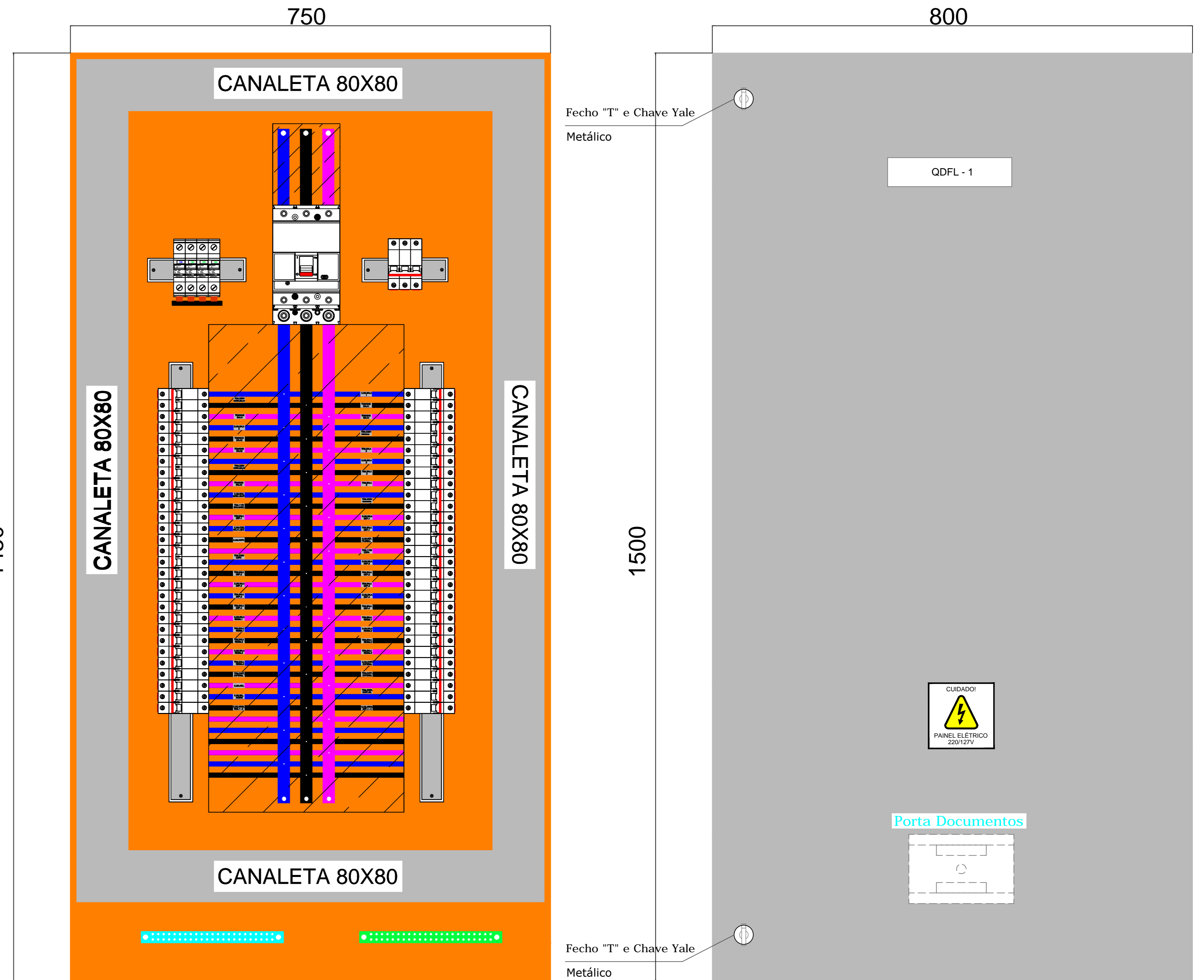
VISTA INTERNA CAIXA DE EMBUTIR 1500X800X250MM
